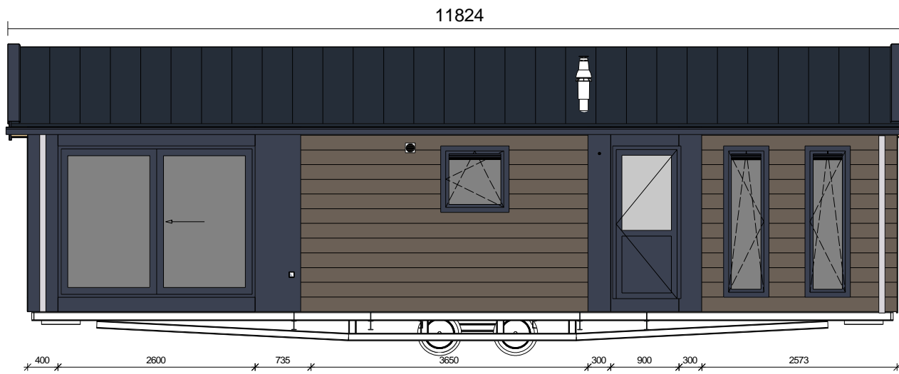
Rechteraanzicht
